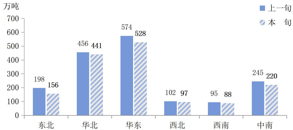
图2 4月下旬六大区域重点统计企业钢材库存情况
